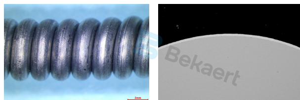
Bezinal® MAX 一倍缠绕及缠绕后的横截面金相
